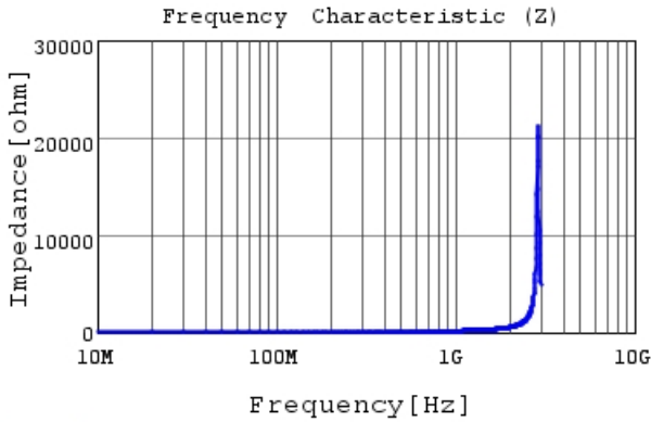
LQG15WZ23NJ02 |Z|
