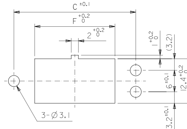
パネル切抜寸法 (参考)
