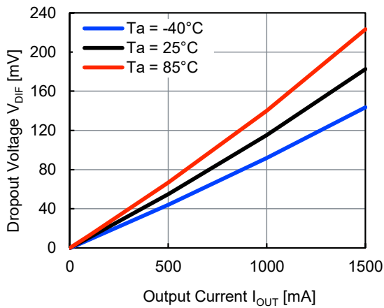
RP120Z121D , CE = V_{BIAS}
