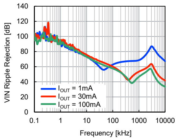
RP120Z121D , V_{IN} = 1.7\text{ V} , V_{ripple} = 0.2\text{V p-p}
