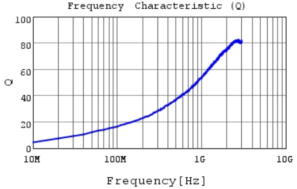
LQG15WZ3N2B02 Q
