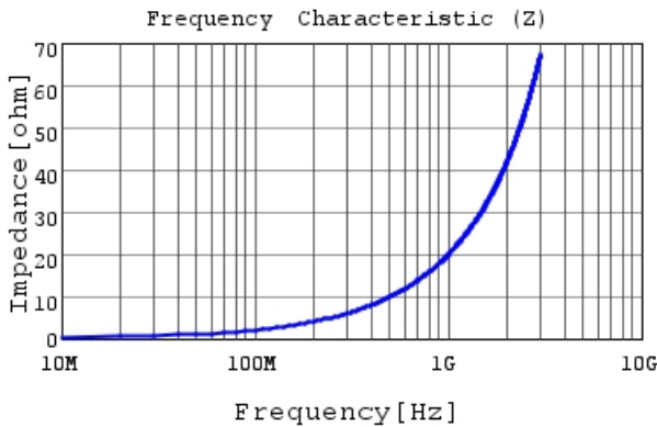
LQG15WZ3N2B02 |Z|
