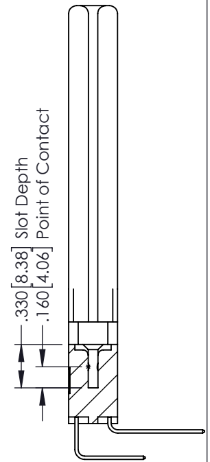
SECTION A-A
