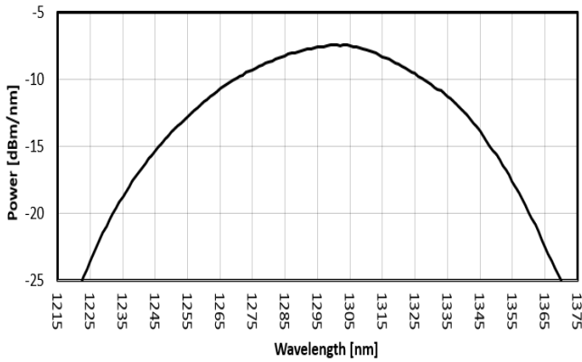
FIG. 1: ISB1 SPECTRUM
