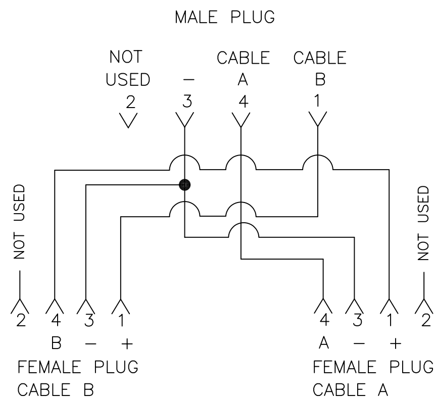
WIRING SCHEMATIC
