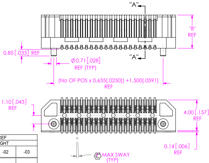
FIG 1 LSS-120-01-XX-DV-A SHOWN
