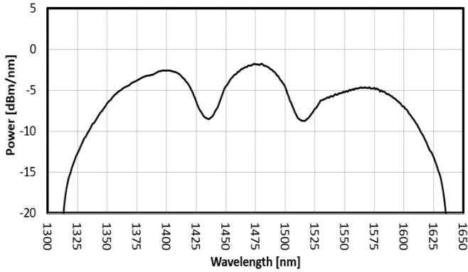
FIG. 1: ISB2 SPECTRUM
