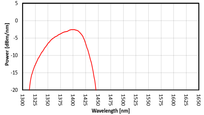
FIG. 4: SLED 3 SPECTRUM
