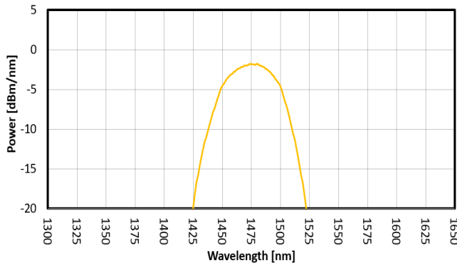
FIG. 3: SLED 2 SPECTRUM
