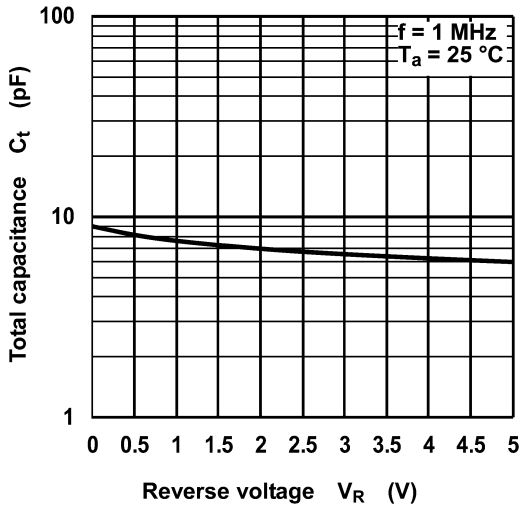
Fig. 8.3 C_t - V_R
