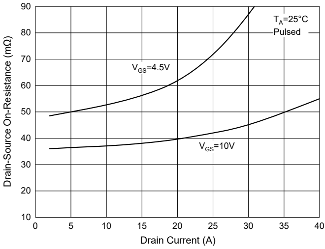
Fig. 1 - R_{DS(ON)} - I_D
