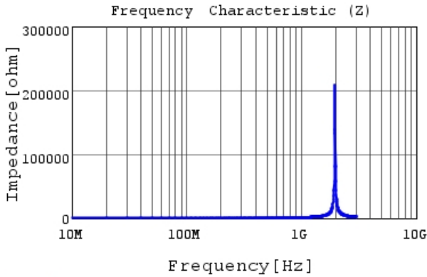
LQW15AWR15J80 |Z|
