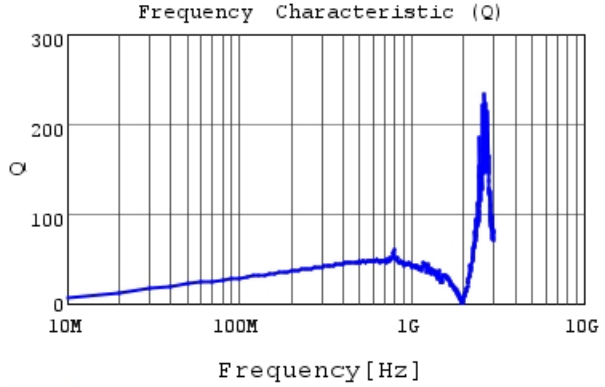
LQW15AWR15J80 Q
