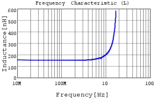
LQW15AWR15J80 L
