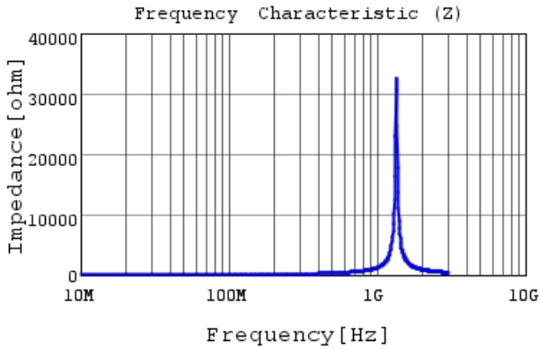
LQG15WH91NH02 |Z|
