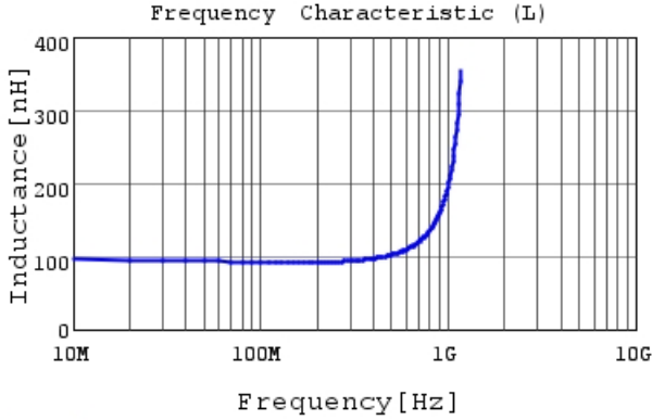
LQG15WH91NH02 L
