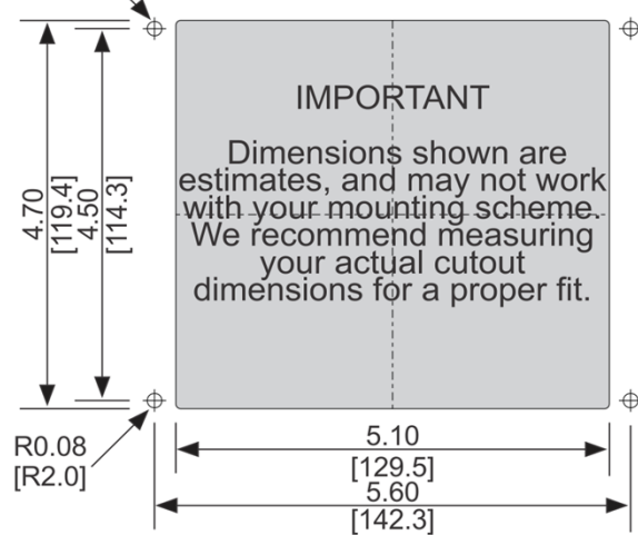
Cutout Dimensions
