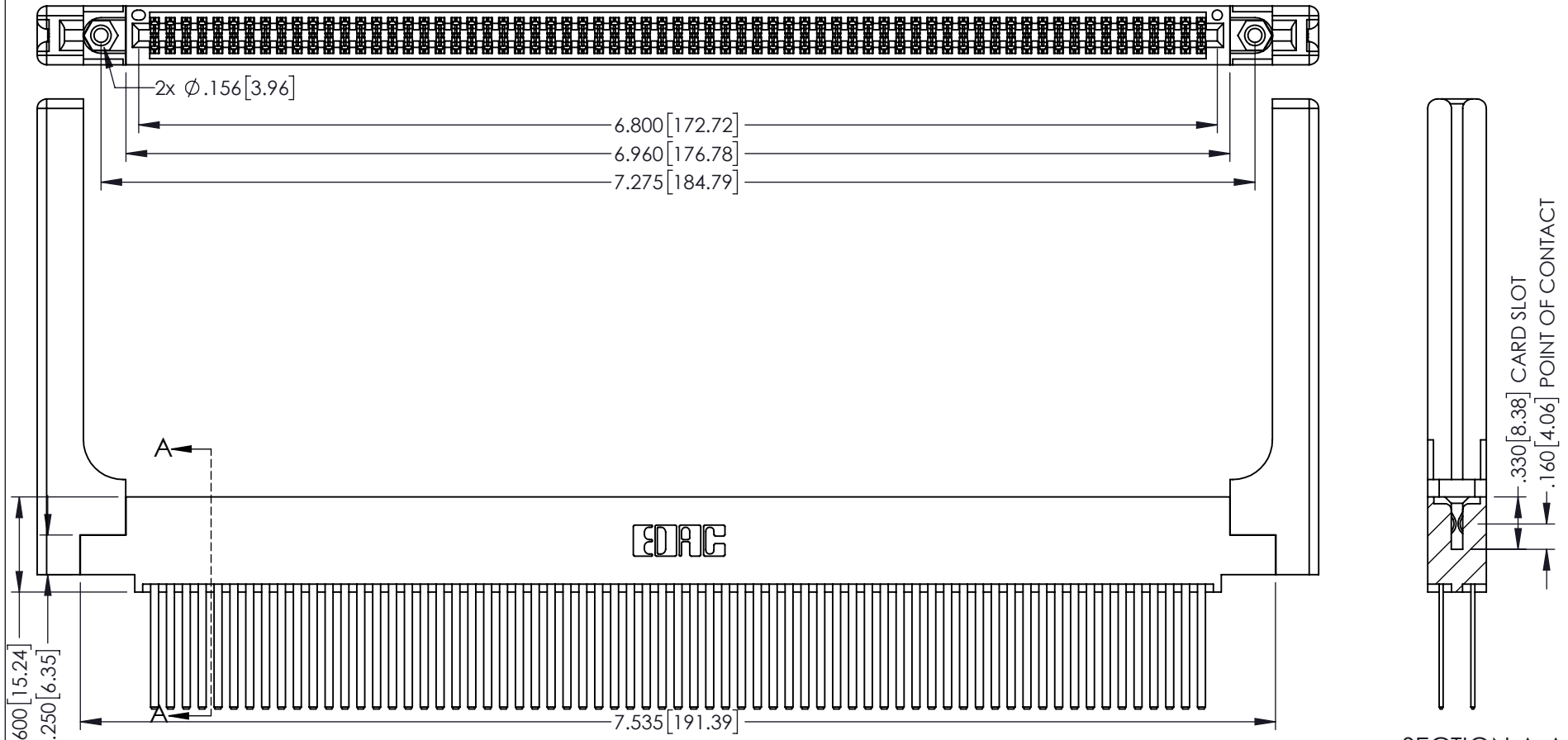
SECTION A-A
