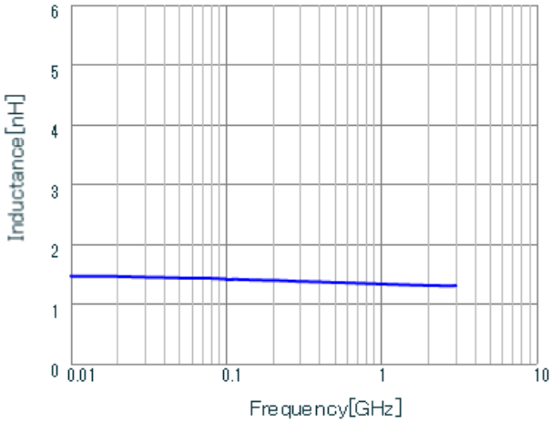
LQP02TN1N4C02 L.
