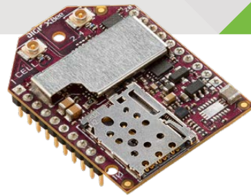
Digi XBee3 Cellular
