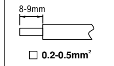
TB2 wiring:
