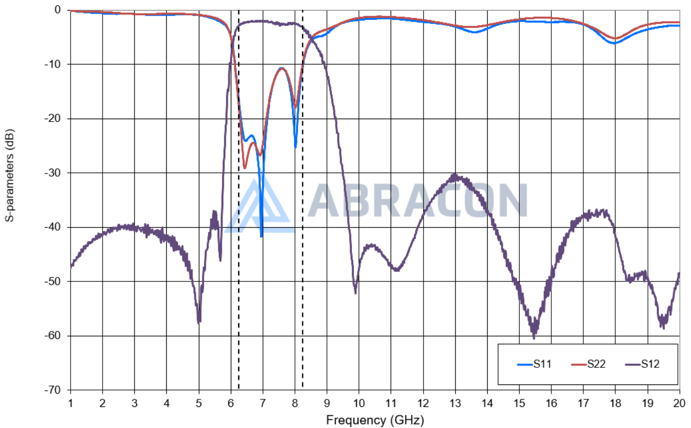
S-parameters
