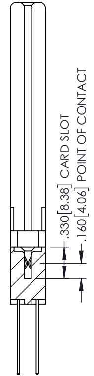
SECTION A-A
