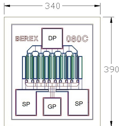
Chip dimensions : 340 X 390 microns Gate pad(GP) : 60 X 60 microns Drain pad(DP) : 70 X 70 microns Source pad(SP) : 70 X 95 microns Chip thickness : 75 microns
