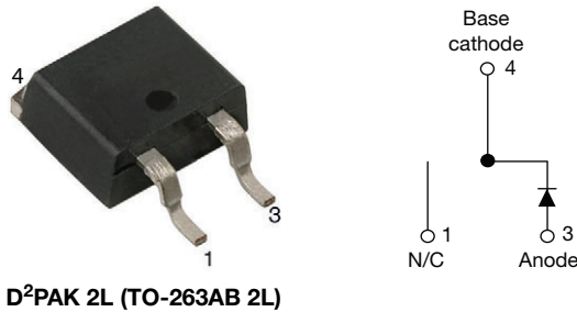
D²PAK 2L (TO-263AB 2L)
