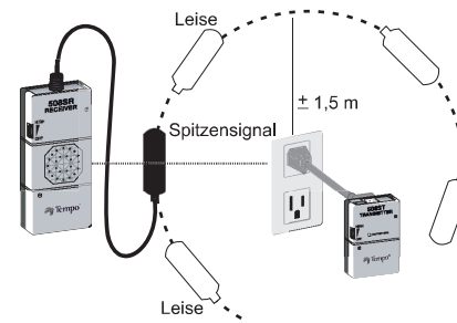
Abb. 03 - Verfolgung von Unterputzleitungen
