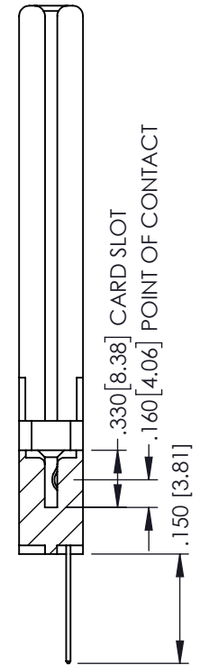
SECTION A-A
