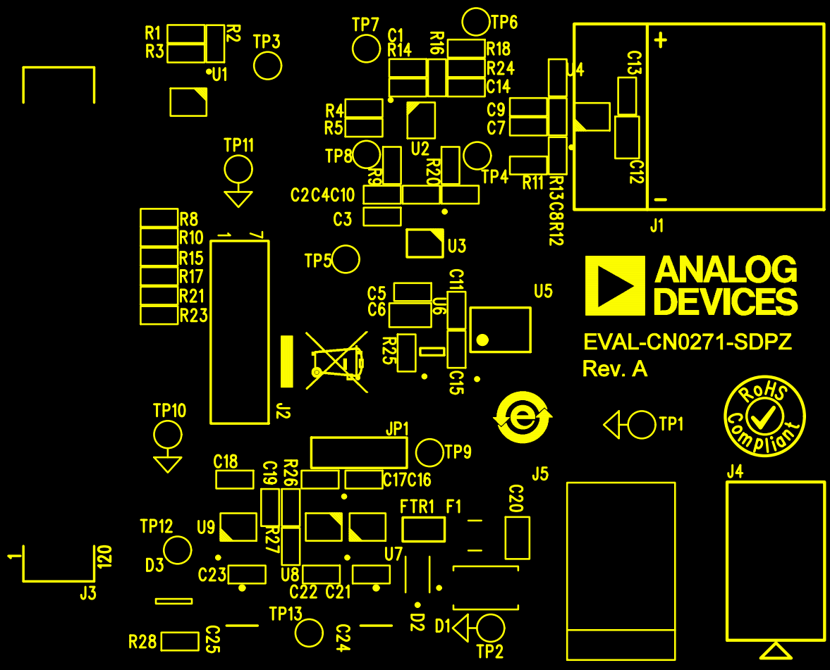
Top Overlay
