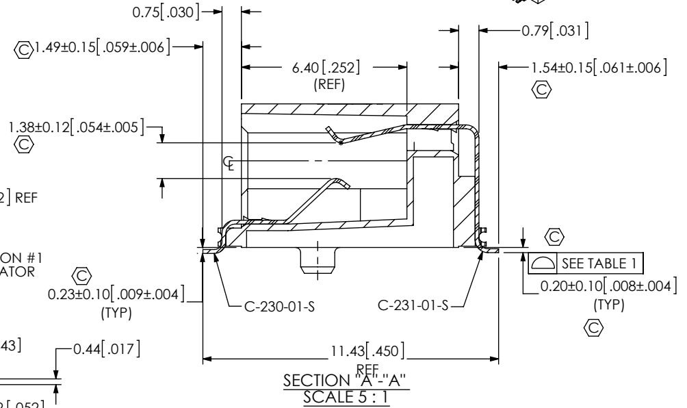
FIG 1 (ER18-031-S-D-RA SHOWN)
