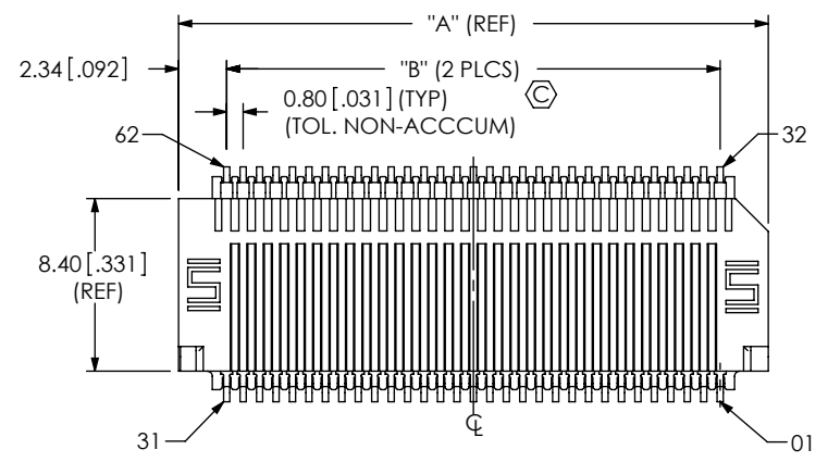
FIG 1 (ER18-031-S-D-RA SHOWN)
