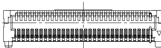
FIG 2 (ER18-031-S-D-RA-K SHOWN)
