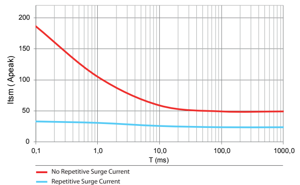
GNAD - 20 A
