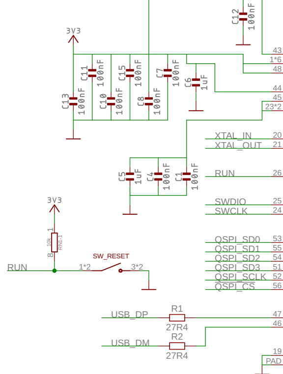
RP2040 MCU
