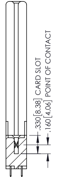
SECTION A-A
