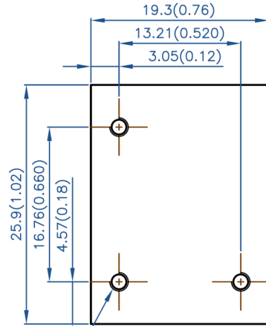
Baseplate Module
