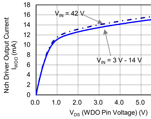
27) WDO Driver Output Current vs. V_{DS}
