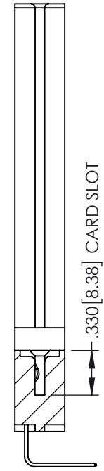
SECTION A-A
