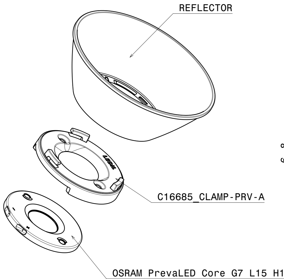
Isometric view Scale: 1:1
