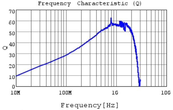
LQW15AW56NG80 Q
