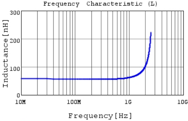
LQW15AW56NG80 L
