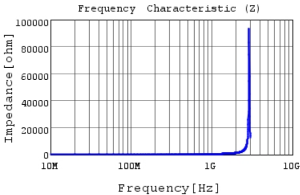
LQW15AW56NG80 |Z|
