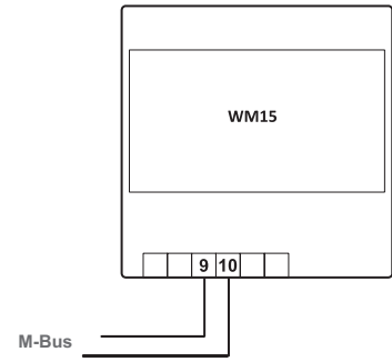
Fig. 16 M-Bus
