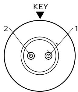
WIRING END W7281-2SG-P-3ES
