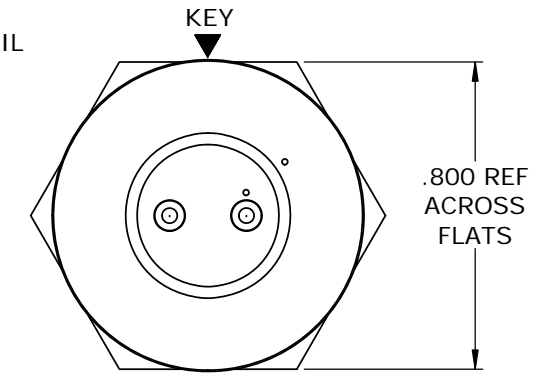
WIRING END W7281-2SG-P-3ES SHOWN
