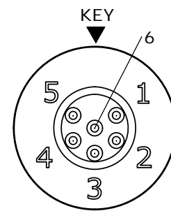
WIRING END W7281-6SG-P-3ES
