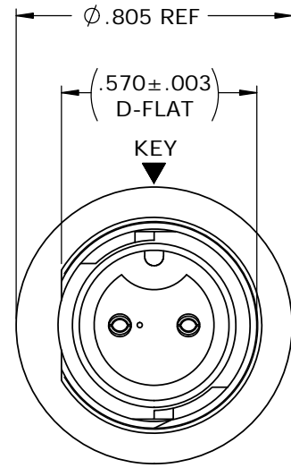
MATING FACE W7281-2SG-P-3ES SHOWN
