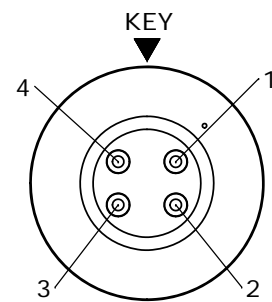
WIRING END W7281-4SG-P-3ES
