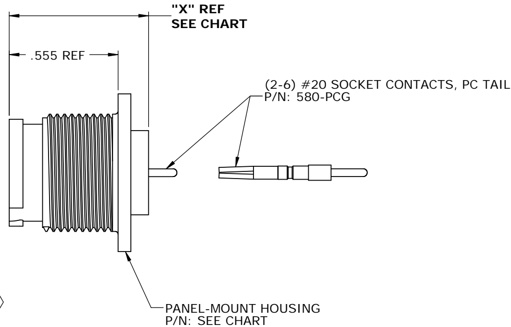
WIRING END W7281-2SG-P-3ES SHOWN
