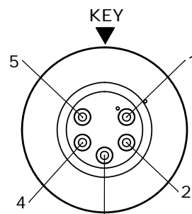
WIRING END W7281-5SG-P-3ES
