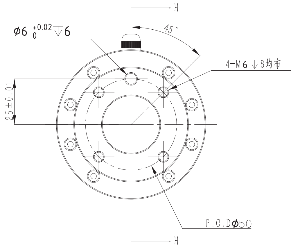
A向视图
