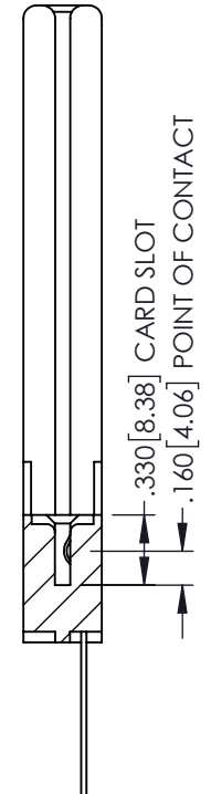
SECTION A-A
