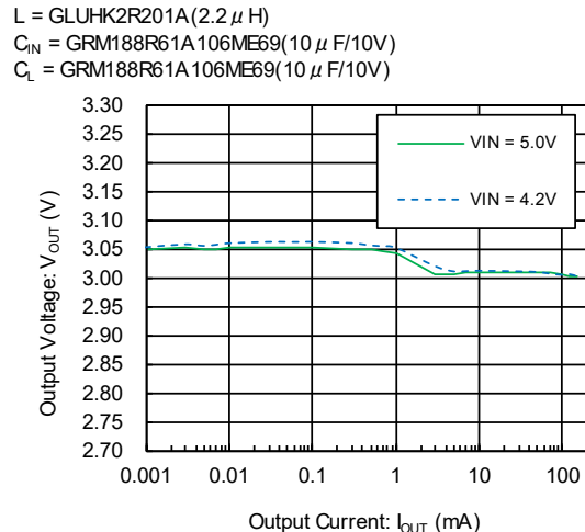
XC9276( V_{OUT}=3.0V )
