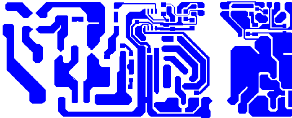
Figure 34. Bottom Layer
