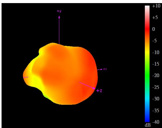
1710MHz
