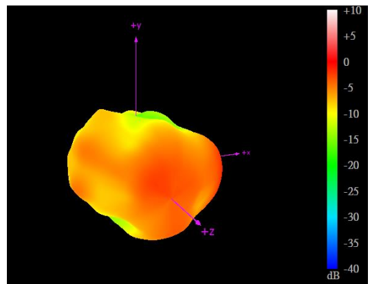
2170MHz
