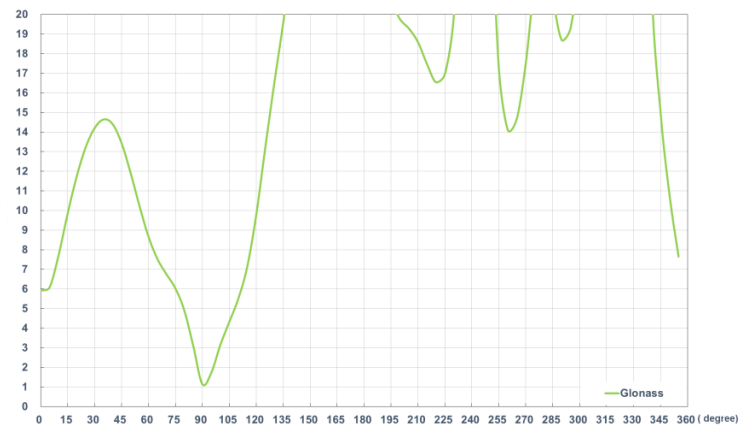
1602MHz
