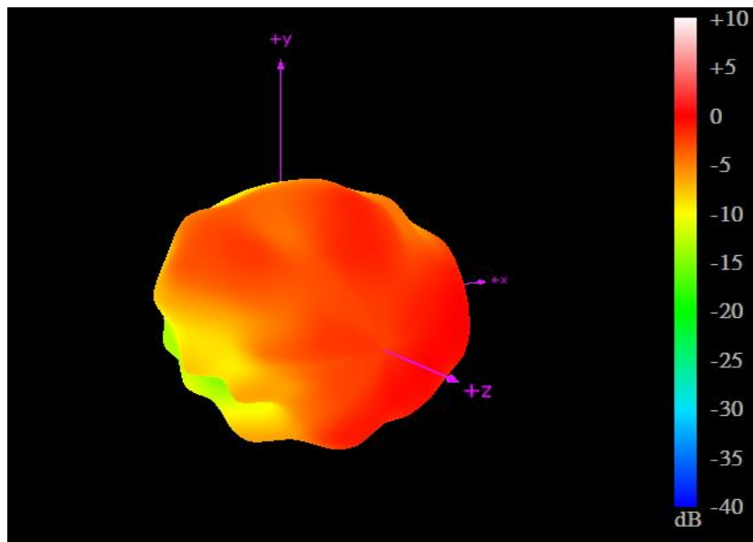
5550MHz
