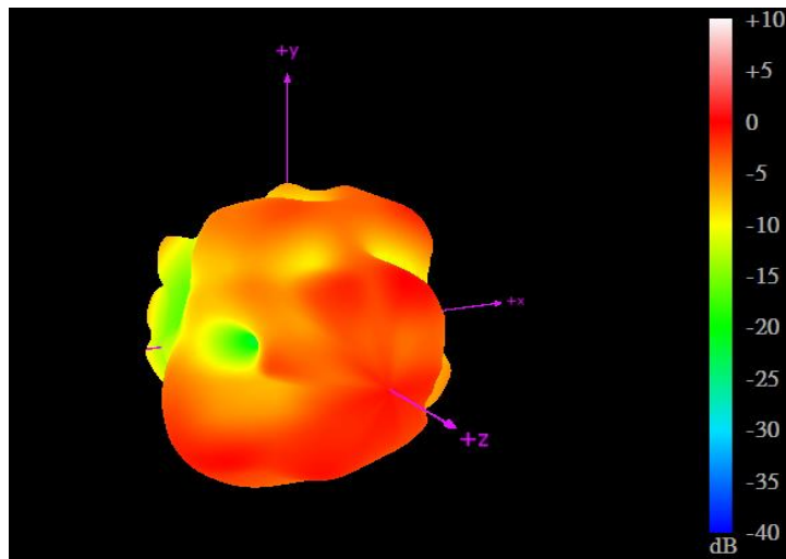
5550MHz
