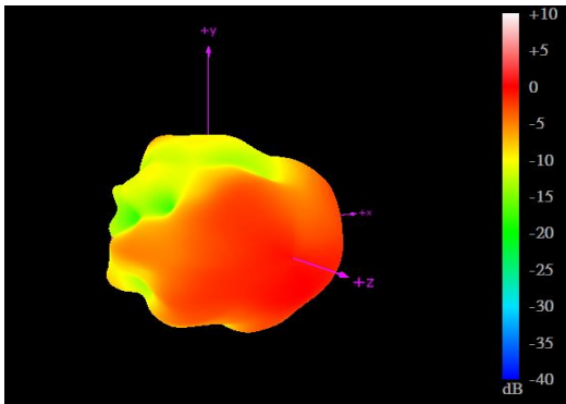
1710MHz
