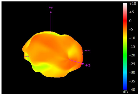
1710MHz
