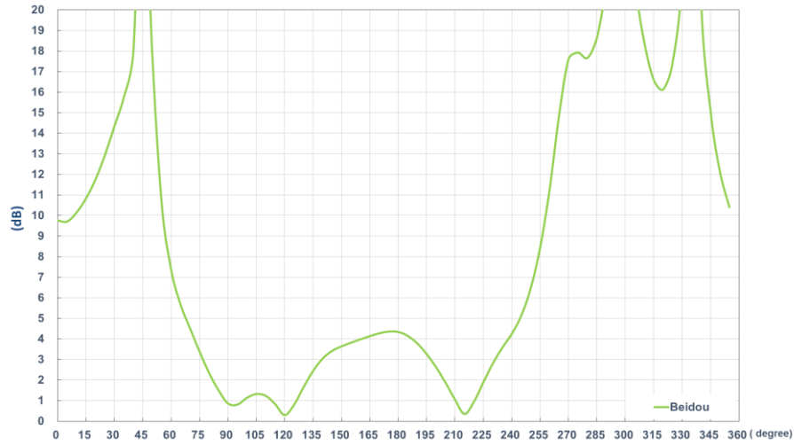
1561MHz
