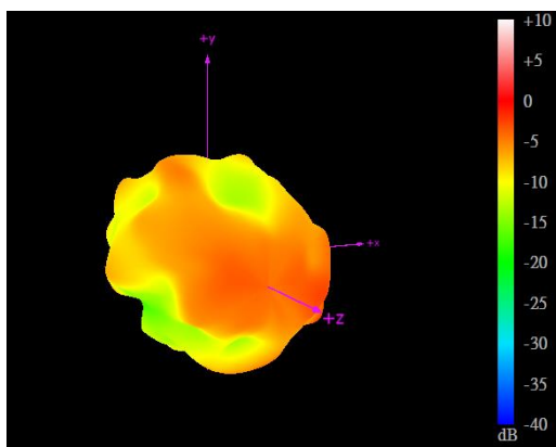
2690MHz
