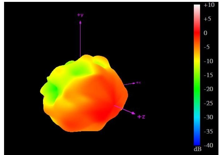
5550MHz
