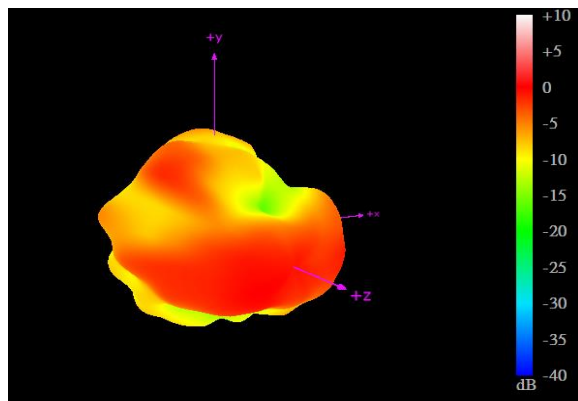
2690MHz
