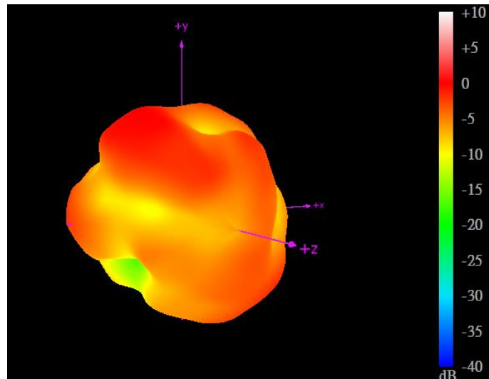
2450MHz
