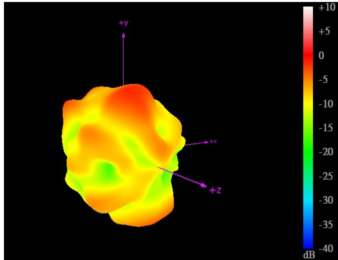
2450MHz
