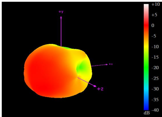
1710MHz
