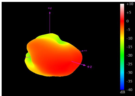
1710MHz
