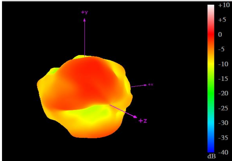
2450MHz
