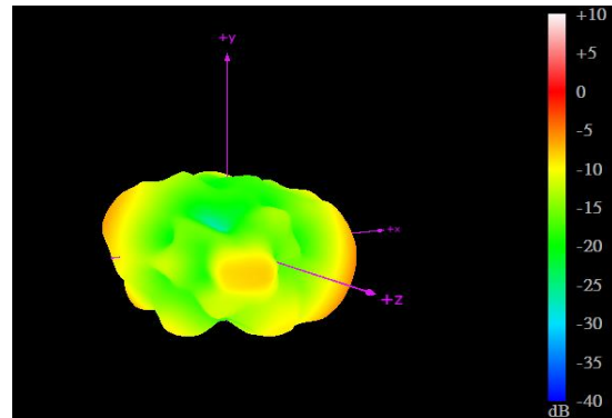
2170MHz
