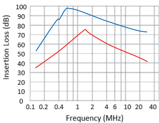
TB1-16A0D0H
