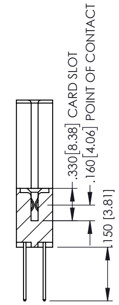
SECTION A-A
