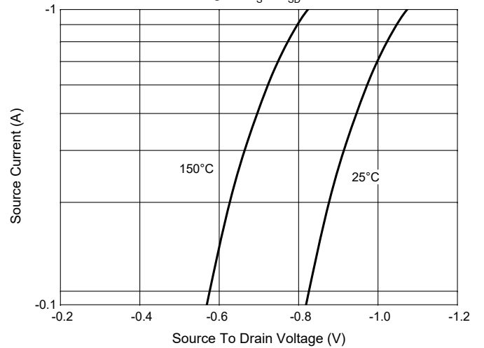
Fig. 4 - I_S - V_{SD}
