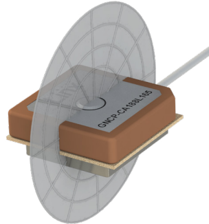
YZ-Plane Gain
