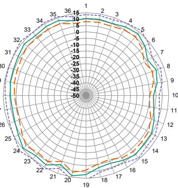
XZ-Plane Gain
