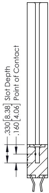
SECTION A-A
