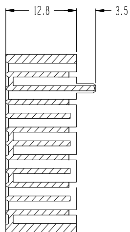
SEZIONE B-B
