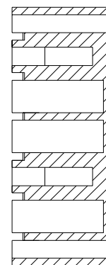
SEZIONE C-C
