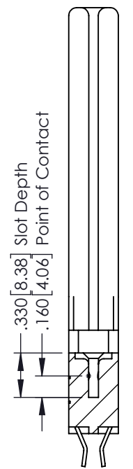
SECTION A-A
