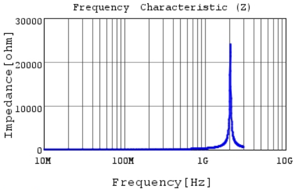
LQG15WH40NJ02 |Z|
