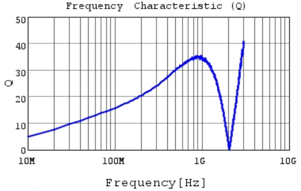
LQG15WH40NJ02 Q
