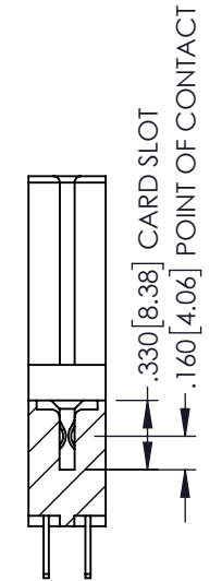
SECTION A-A
